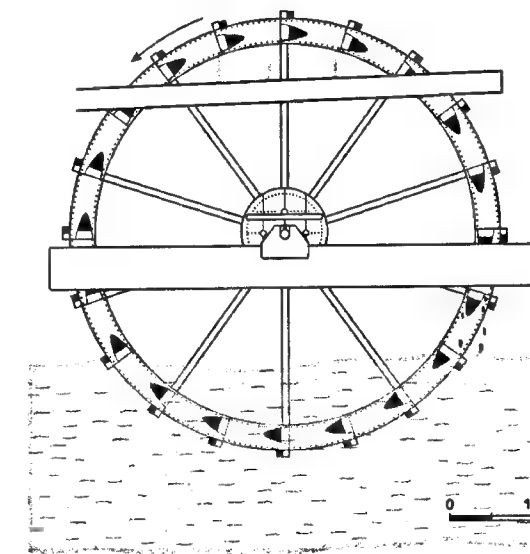
Wasserheberad; aus Dolaucothi, Wales (Rekonstruktion).
